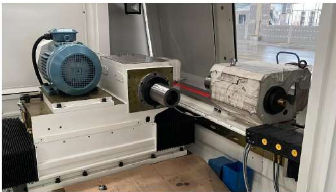
Станок циркулярной шлифовки
