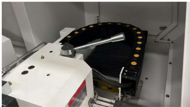
Внутренняя камера станка
