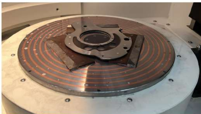
Обрабатываемые детали на станке серии SGR
