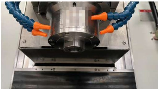
Нижняя часть вертикального шпинделя станка [redacted]
